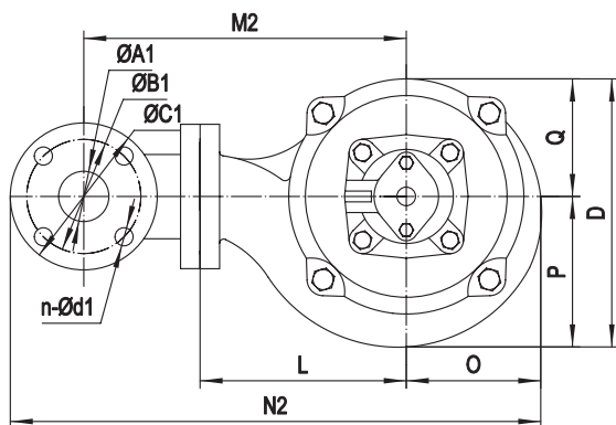
Размеры напорного патрубка насоса
